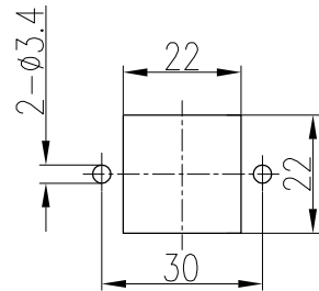
面板开孔图
